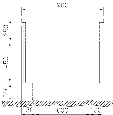
Zij aanzicht
